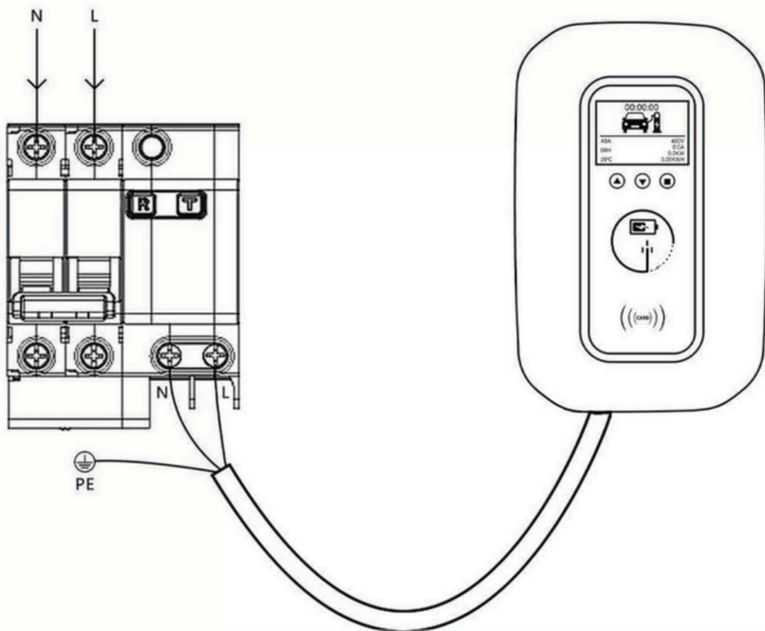
Diagrama de instalación de cableado monofásico
